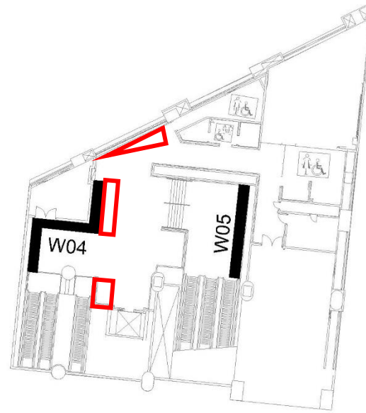
3F連通道層平面圖
